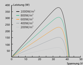
Leistung-Spannung-Kennlinie (380W)
