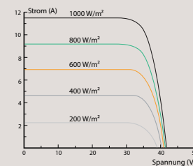
Strom-Spannungs-Kennlinie (380 W)
