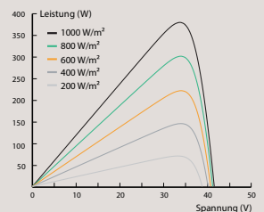
Leistung-Spannungs-Kennlinie (380 W)
